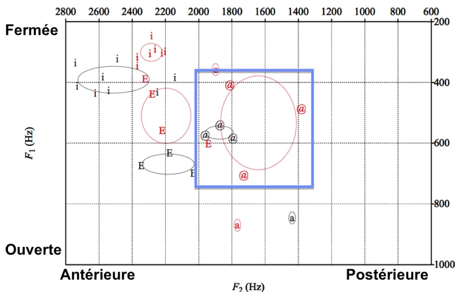
Figure 2 : triangles vocaux chez une native britannique (noir) et une apprenante d'ALE d'origine française (rouge) produisant la phrase : "This money won't buy anything, he said, it's Egyptian". Les ellipses représentent un écart-type de la production moyenne de chaque voyelle, montrant leur dispersion. Le rectangle bleu représente la zone des voyelles centrales, beaucoup plus dispersée chez l'apprenante francophone.
