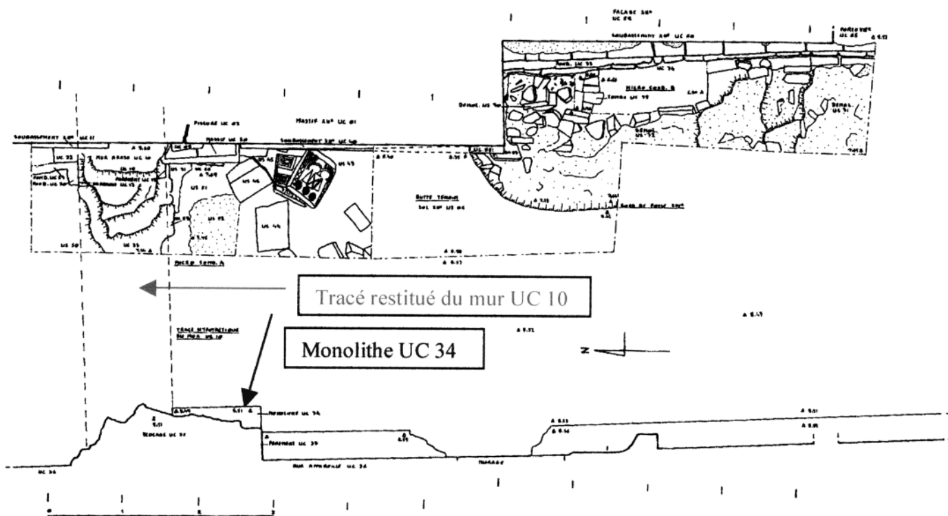
Fig. 8 - Saint-Gilles-du-Gard, ancienne abbatale, plan du sondage réalisé en 2004 au pied du soubassement de la façade occidentale (C. Markiewicz d'après Markiewicz 2004, p. 17, fig. 17).
