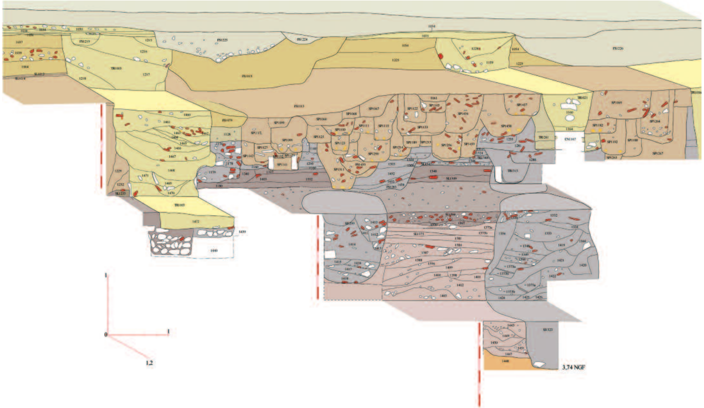
Fig. 14 - Saint-Gilles-du-Gard, les fouilles du cloître en 2010, coupe stratigraphique axonométrique sud-nord (L. Buffat, A. Masbernat-Buffat, 2010-2011. D'après Masbernat-Buffat, Buffat, Hartmann-Virnich, Legrand-Garnotel, Schneider, Chazottes 2012, p. 115, annexe 4).
