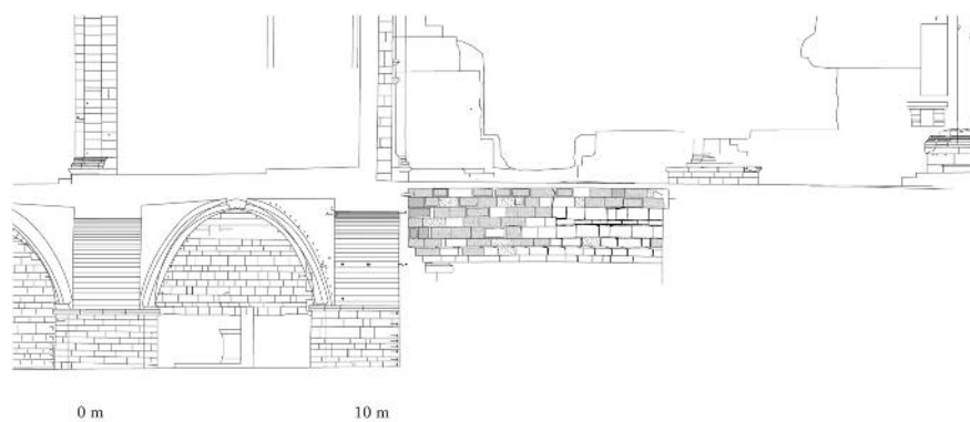
Fig. 1 - Saint-Gilles-du-Gard, ancienne abbatale, coupe longitudinale avec élévation partielle du soubassement du mur gouttereau nord, vectorisé d'après le relevé réalisé en 1980 par l'Association d'Histoire et d'Archéologie de Saint-Gilles (relevé H. Hansen, D.A.O. L. Maggiori).
