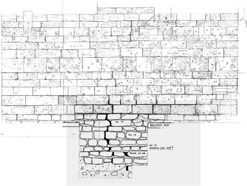
Fig. 10 - Saint-Gilles-du-Gard, crypte, mur gouttereau sud, parement intérieur, quatrième travée. Relevé pierre-à-pierre (H. Hansen) intégrant le relevé des fondations dégagées en 2004 (C. Markiewicz d'après Markiewicz 2004, p. 57, fig. 53).
