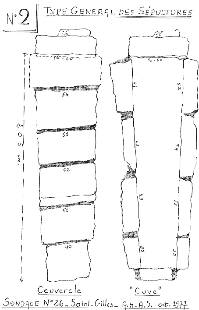
Fig. 5 - Saint-Gilles-du-Gard, ancienne abbatale, schéma-type des sépultures à coffrage de pierre dégagées dans le bras nord du transept et dans le collatéral nord du chevet (sondage 26). R. Jeolas, 26 octobre 1977 (Archives de l'Association d'Histoire et d'Archéologie de Saint-Gilles).
