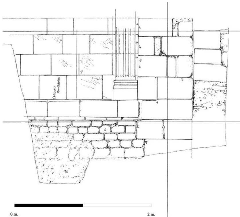
Fig. 11 - Saint-Gilles-du-Gard, bâtiment claustral sud, façade nord, relevé pierre-à-pierre de la travée dégagée lors du sondage 1 (sondages C. Markiewicz, 2009) [H. Hansen, 2009].
