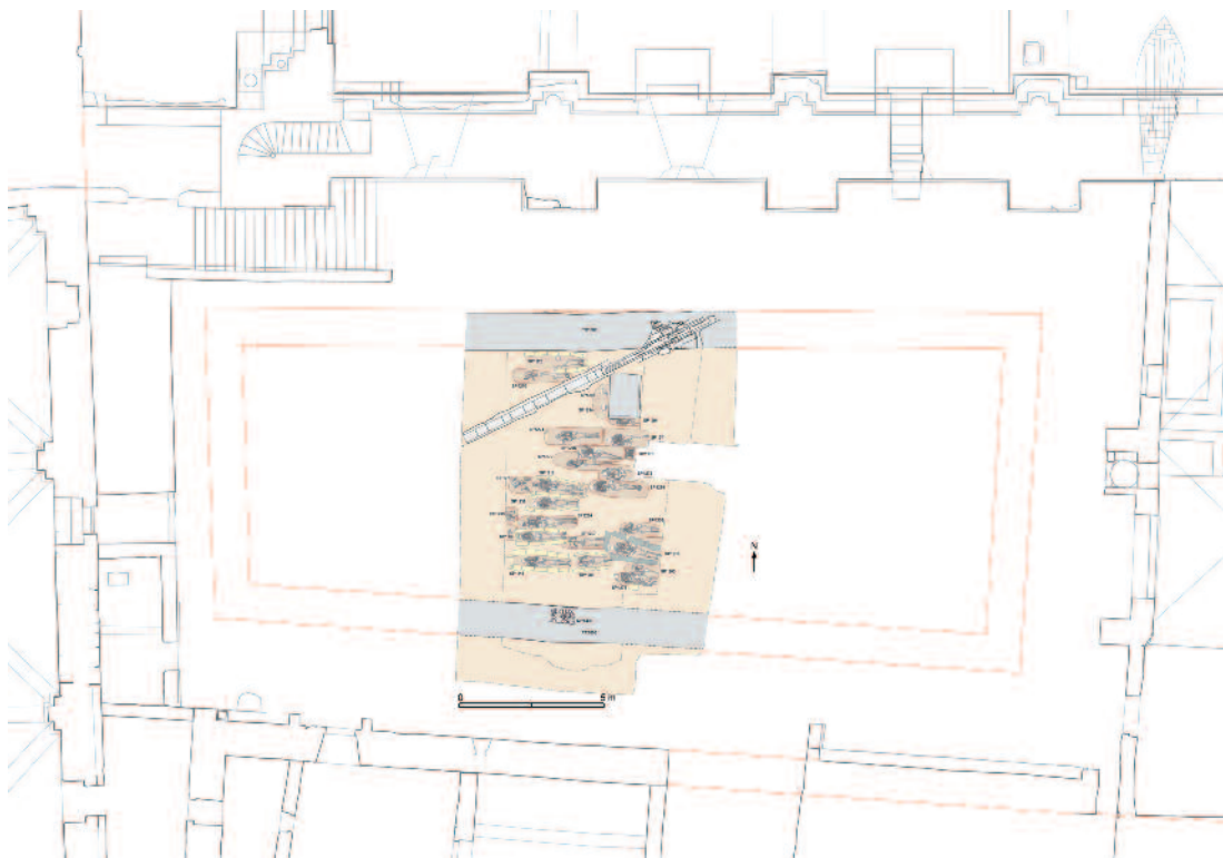
Fig. 12 - Saint-Gilles-du-Gard, plan de l'espace claustral avec l'emprise de la fouille de 2010 et l'emplacement restituée des murs-bahuts des galeries dans leur second état (H. Hansen, 2010 ; L. Buffat, A. Masbernat-Buffat, 2010-2011. D'après Masbernat-Buffat, Buffat, Hartmann-Virnich, Legrand-Garnotel, Schneider, Chazottes 2012, p. 95, fig. 7.06).
