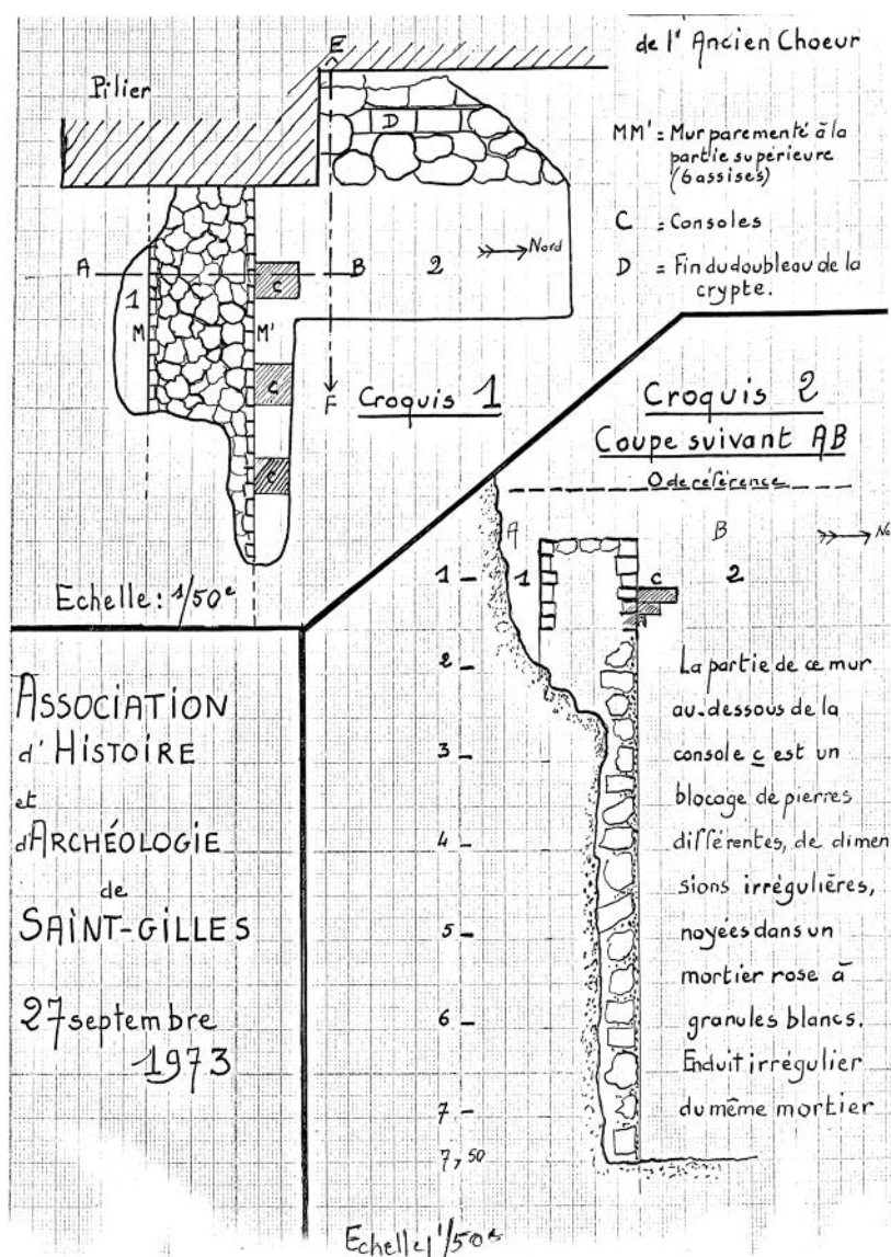
Fig. 2 - Saint-Gilles-du-Gard, ancienne abbatale, coupe et plan schématiques du mur est-ouest dégagé sous la croisée du transept, R. Jeolas, septembre 1973 (Archives de l'Association d'Histoire et d'Archéologie de Saint-Gilles).
