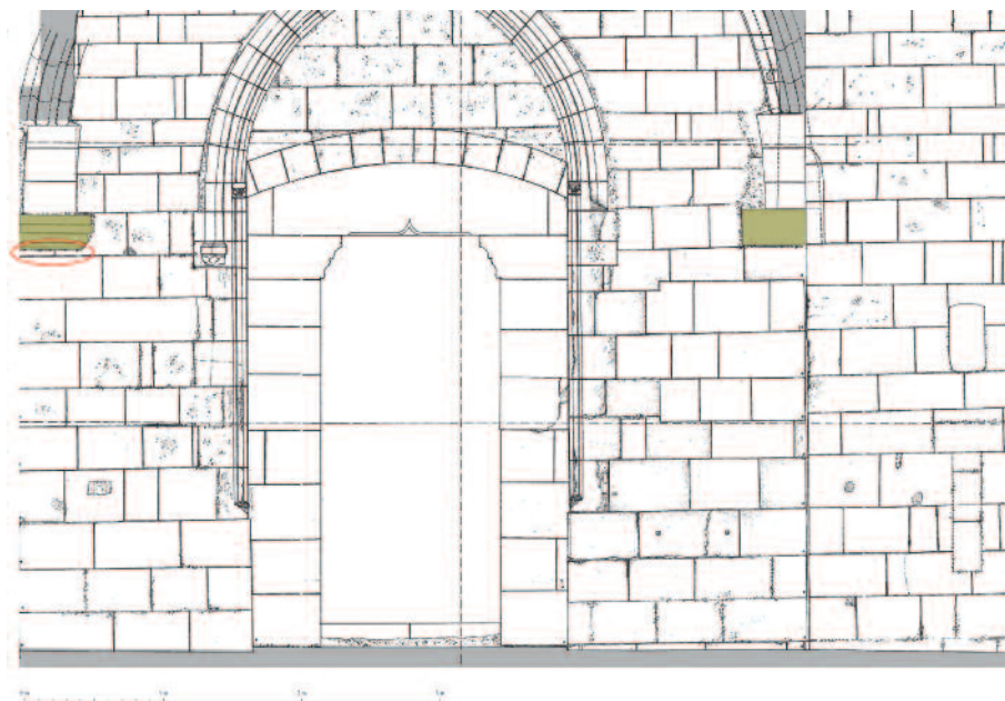
Fig.15 - Saint-Gilles-du-Gard, ancienne abbatale, revers de la façade occidentale, parement du collatéral sud : corrections au niveau avec indication des consoles (H. Hansen, 1999-2002).
