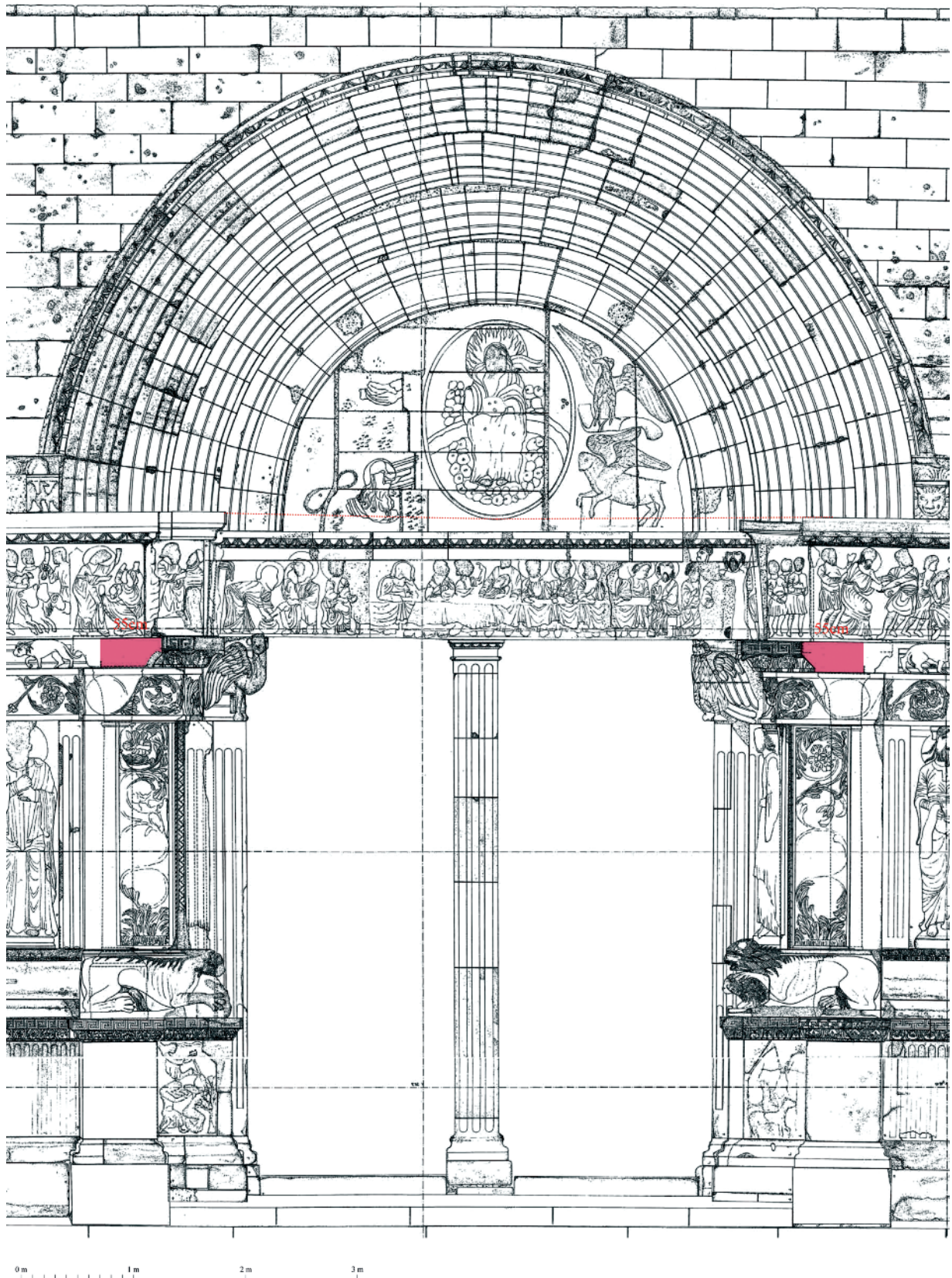
Fig. 25b - Saint-Gilles-du-Gard, ancienne abbatale, façade occidentale. Largeur de l'emplacement prévu pour l'insertion des tailloirs nord et sud du portail central (H. Hansen, 1999-2002).
