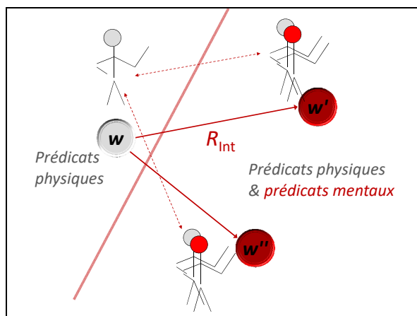
Fig.5. Sphère physicaliste et sphère intentionnelle
