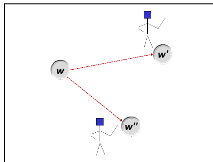
Fig.4. Croyance de objecto
