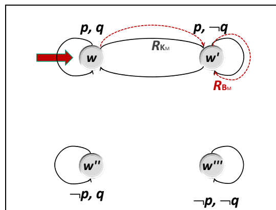
Fig.1. Possibilités aléthiques, épistémiques et doxastiques
