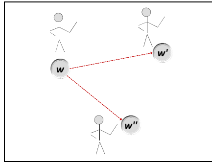
Fig.3. Croyance de re
