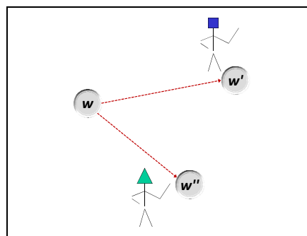
Fig.2. Croyance de dicto
