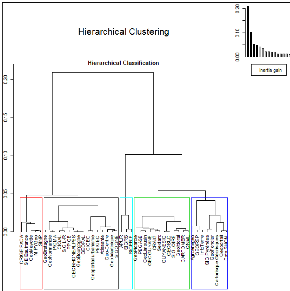
Figure 11. Arbre hiérarchique
