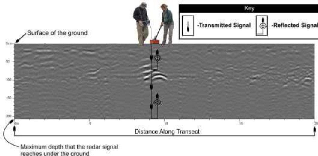
Figure 19 : schéma de la collecte d'un transect GPR et la réflexion de l'énergie GPR par une cible souterraine (Sullivan & Connell, 2012)
