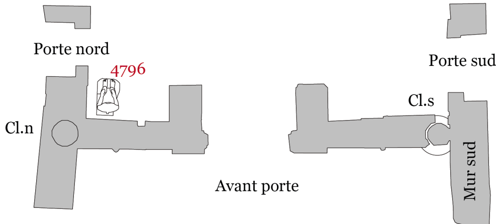
Cour axiale du V e pylône, avant-porte du VI e pylône, plan schématique.
