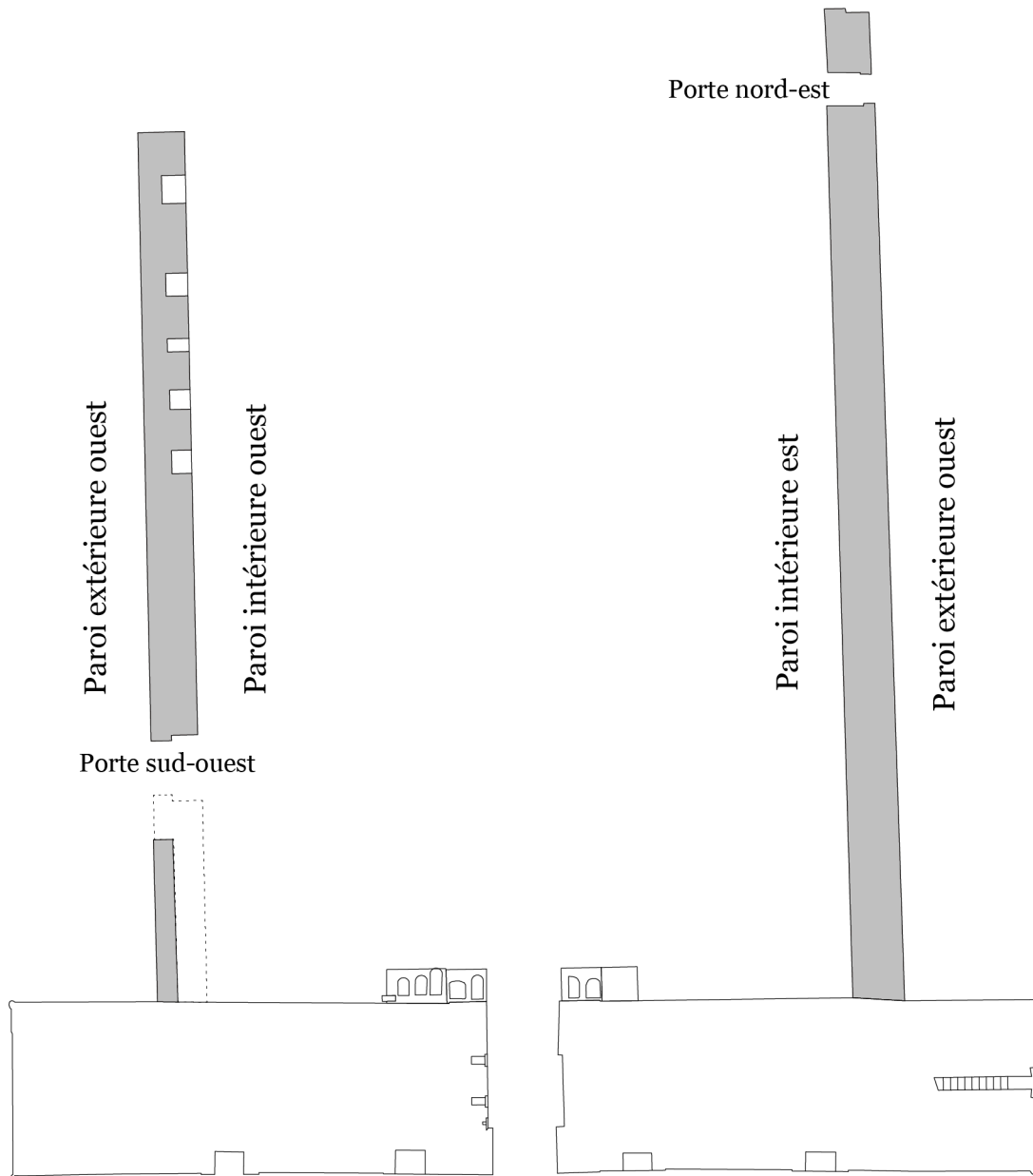
Cour du VII e pylône - « Cour de la cachette », plan schématique.
