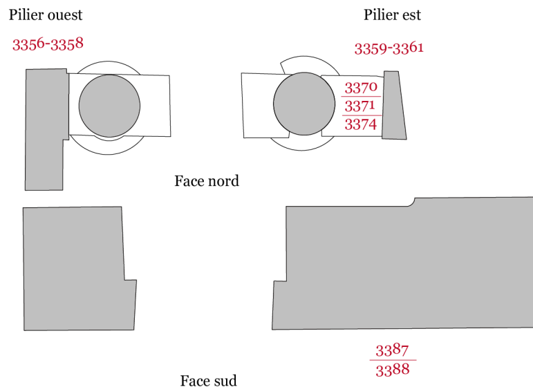
Porte bubastide Sud, plan schématique.
