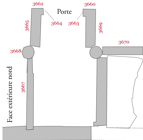
Chapelle au nord de l'obélisque, plan schématique.
