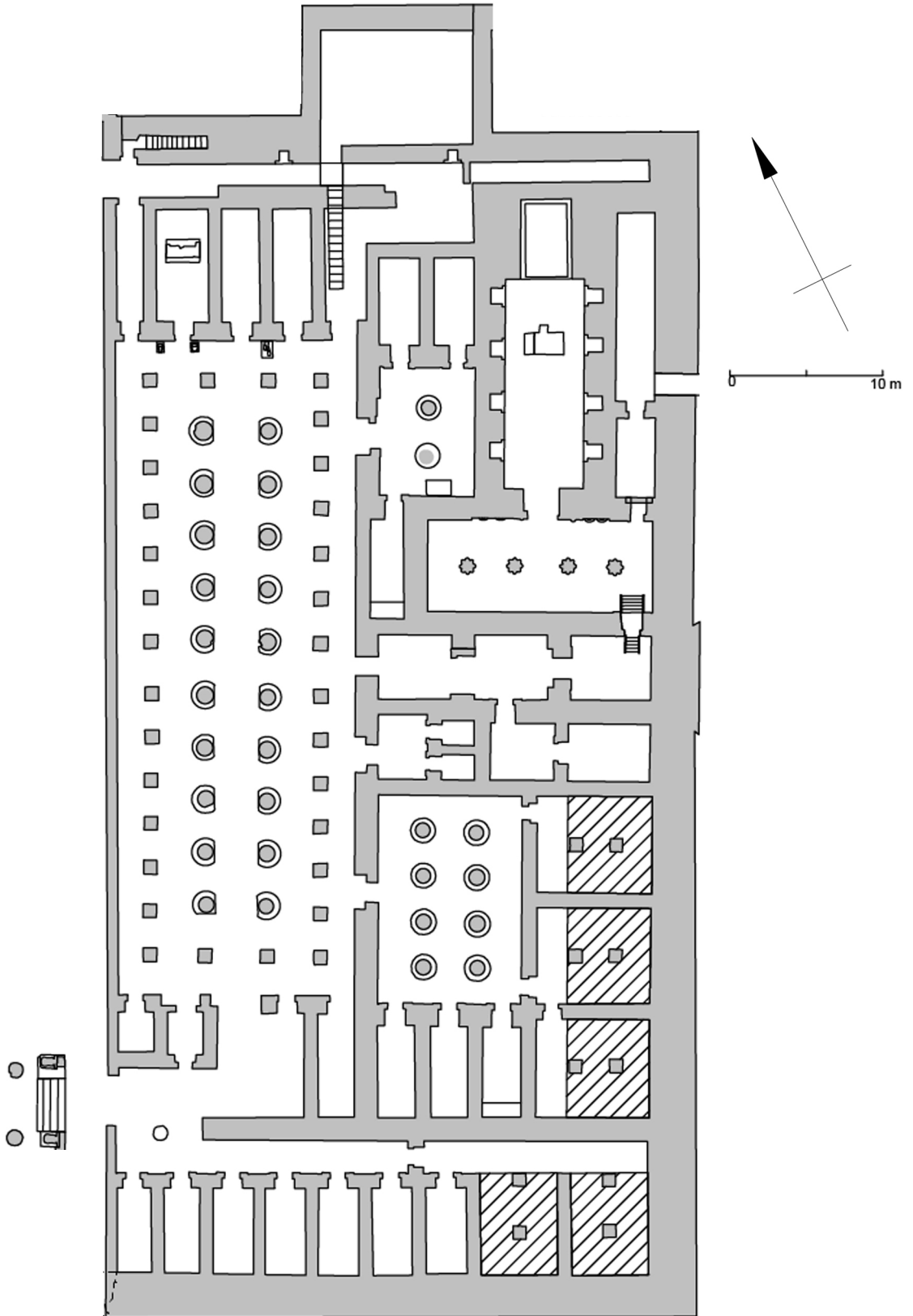
Akh-menou, plan schématique.
