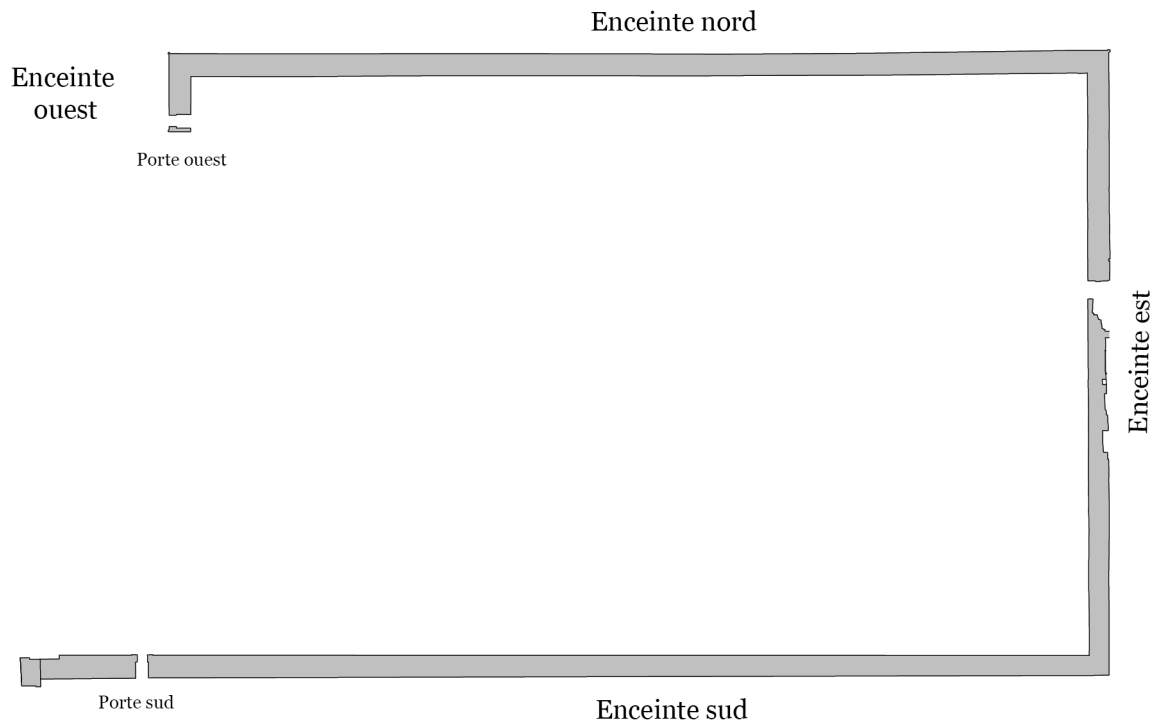
Mur extérieur de Thoutmosis III, plan schématique.
