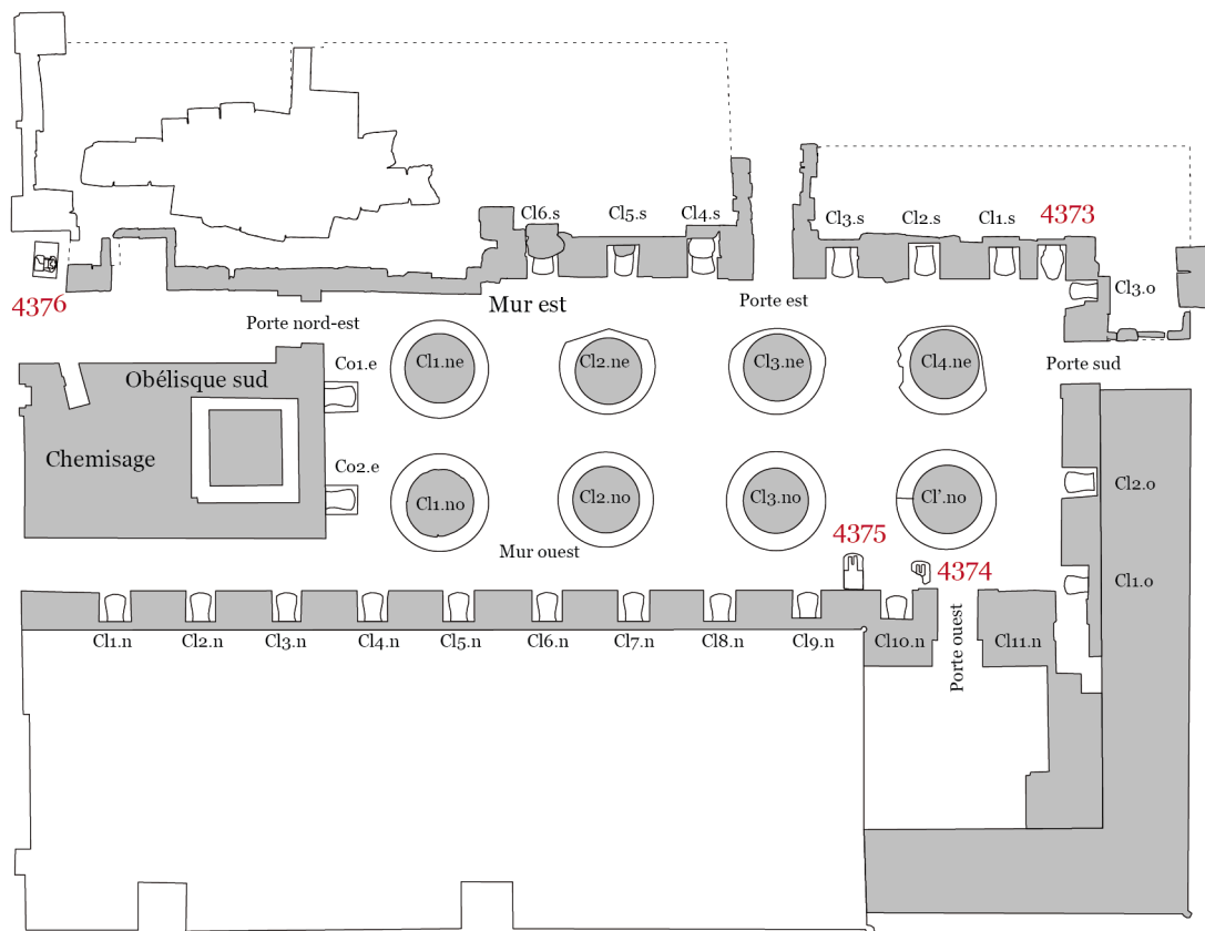
Cour sud du IV e pylône, plan schématique.
