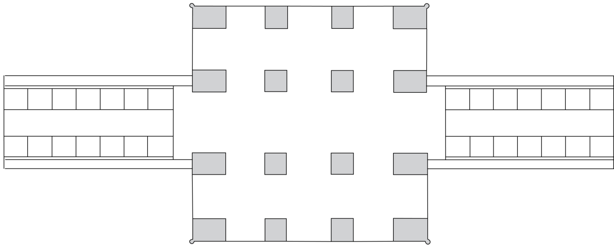
Chapelle blanche, plan schématique.
