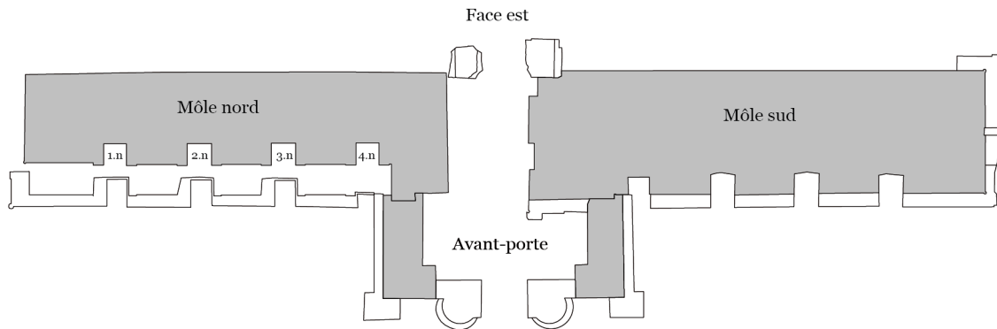
III e pylône, plan schématique.
