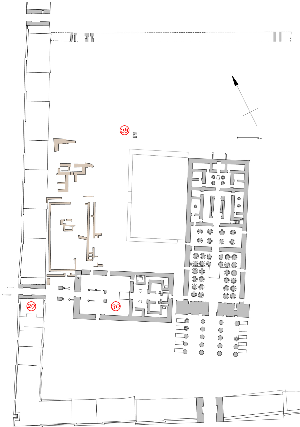
Zone sud ouest, plan schématique.
