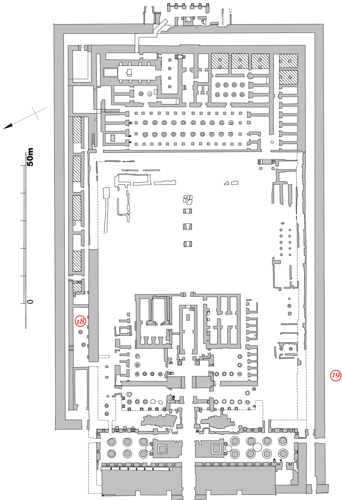
Mur extérieur de Thoutmosis III, plan schématique.
