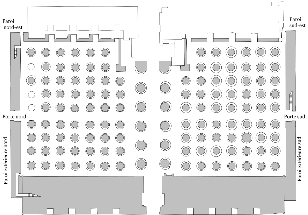
Salle hypostyle, plan schématique.
