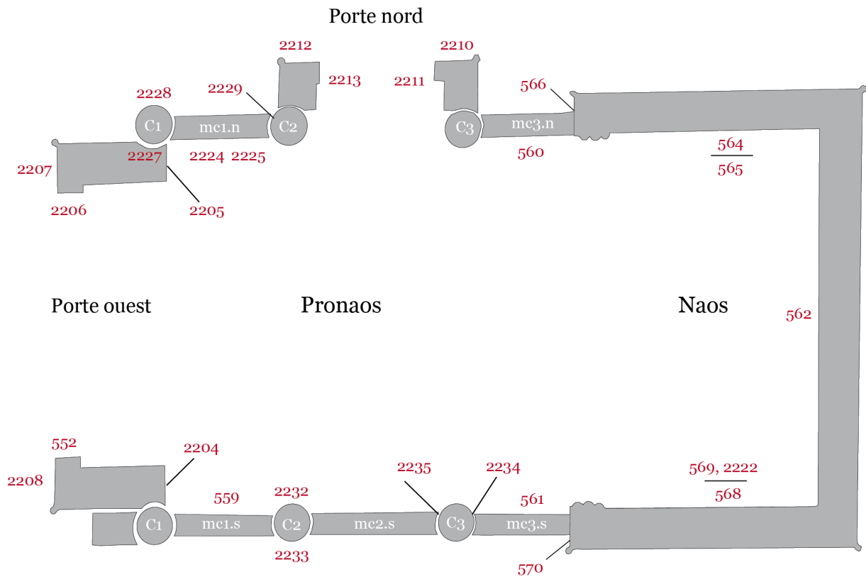
Chapelle d'Achôris, plan schématique.
