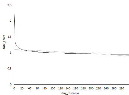
FIGURE 1 - Courbe de la fonction score_date
