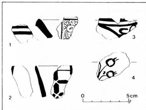
Fig. 4 - Céramiques à pâte siliceuse et décor polychrome sous glaçure incolore (1. séries de 3 points pour le vert, pointillé pour le bleu; 2. pointillé pour le bleu, pointillé plus serré pour le brun; 3. pointillé plus aéré pour le bleu turquoise; 4. pointillé pour le rouge brun).
