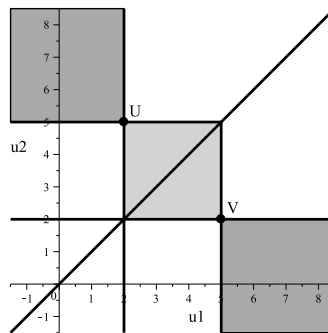
(d) Leximin-Antileximax
