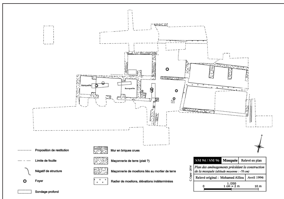
Figure 9: Plan de la structure domestique midraride dite “maison à alcôves” (d’après les relevés du MAPS)
