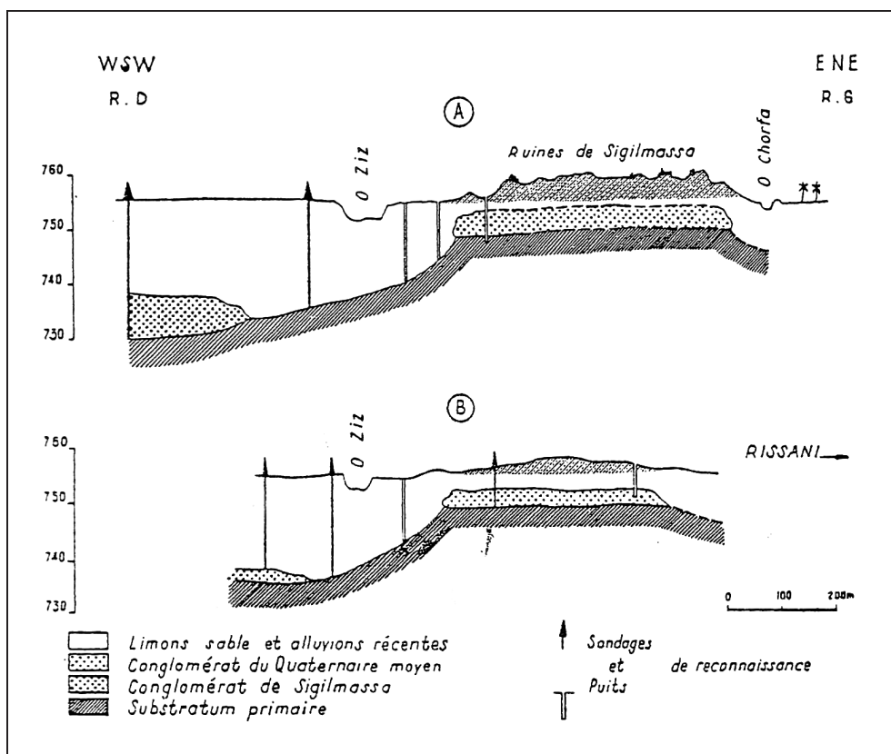
Figure 3: Schémas en coupe du profil géologique du substrat sous le tell archéologique de Sijilmāsa: A – au niveau de la “citadelle” (moitié nord du site); B – au niveau de la route asphaltée (entre du site) (source: Jean Margat, “Note sur la morphologie du site”)
