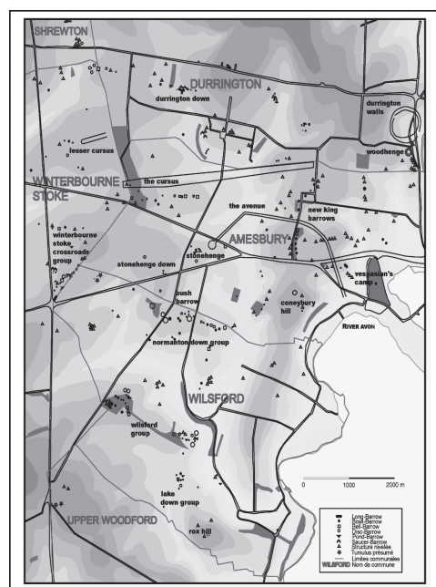
Fig. 3 - zone autour de Stonehenge (0 partir de Cunliffe et al)
