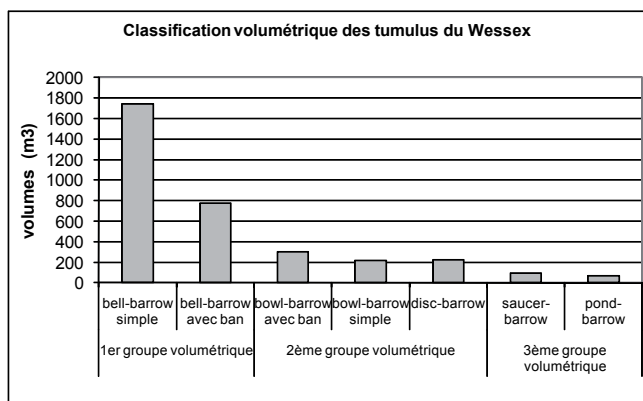
Fig. 2- Classification volumétrique des tumulus du Wessex
