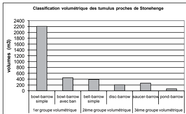
Fig. 4- Classes volumétriques obtenues à proximité de Stonehenge.
