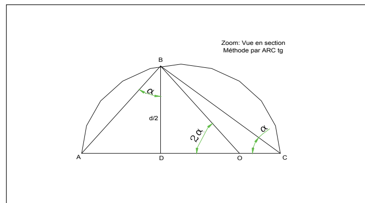
Fig. 6 - Méthode de calcul
