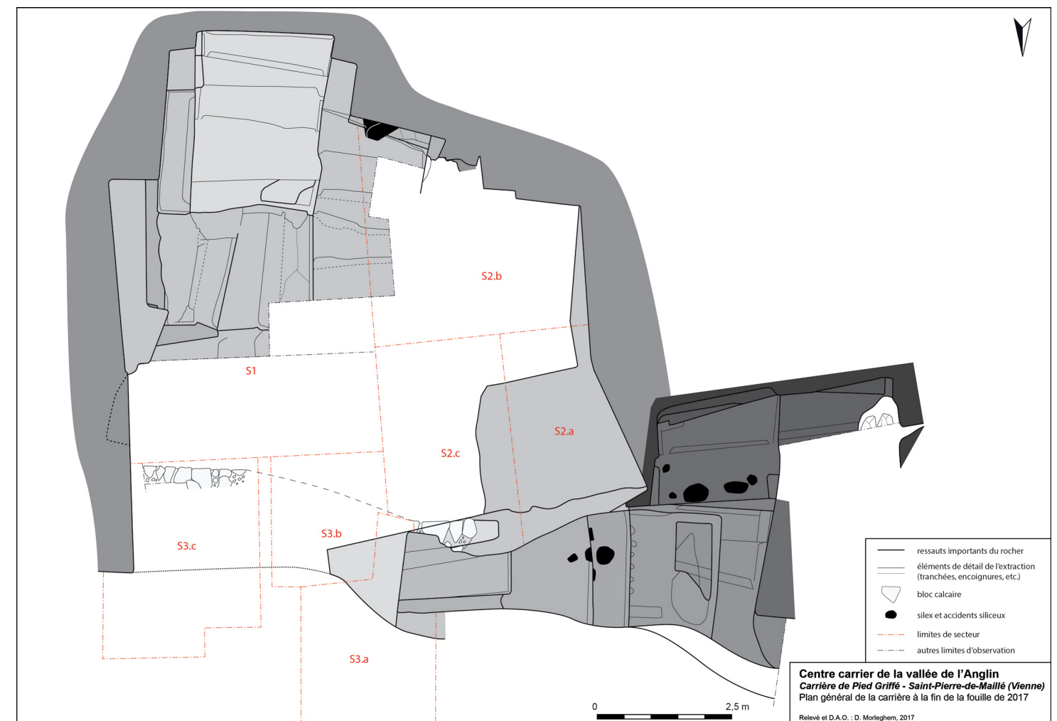
Fig. 4 - Plan général de la carrière (état 2017)
