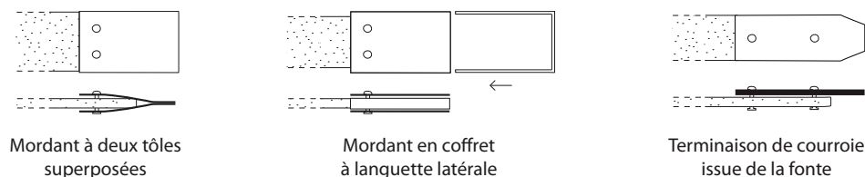
Quelques types de mordants et terminaisons de courroie
