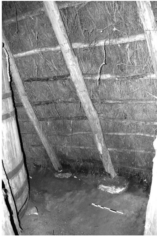
Fig. 31 Ambillou, « La Giberdière ». Pieds des chevrons de la croupe, en appui sur des pierres plates (cl. F. É.).
