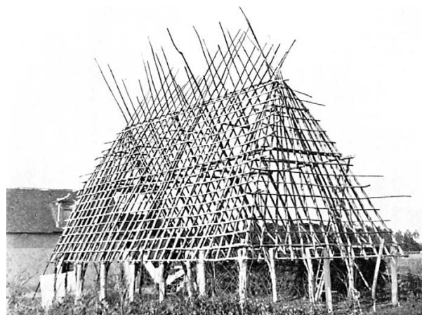
Fig. 58 Fixation du lattis (STEMMERMANN 1942).
