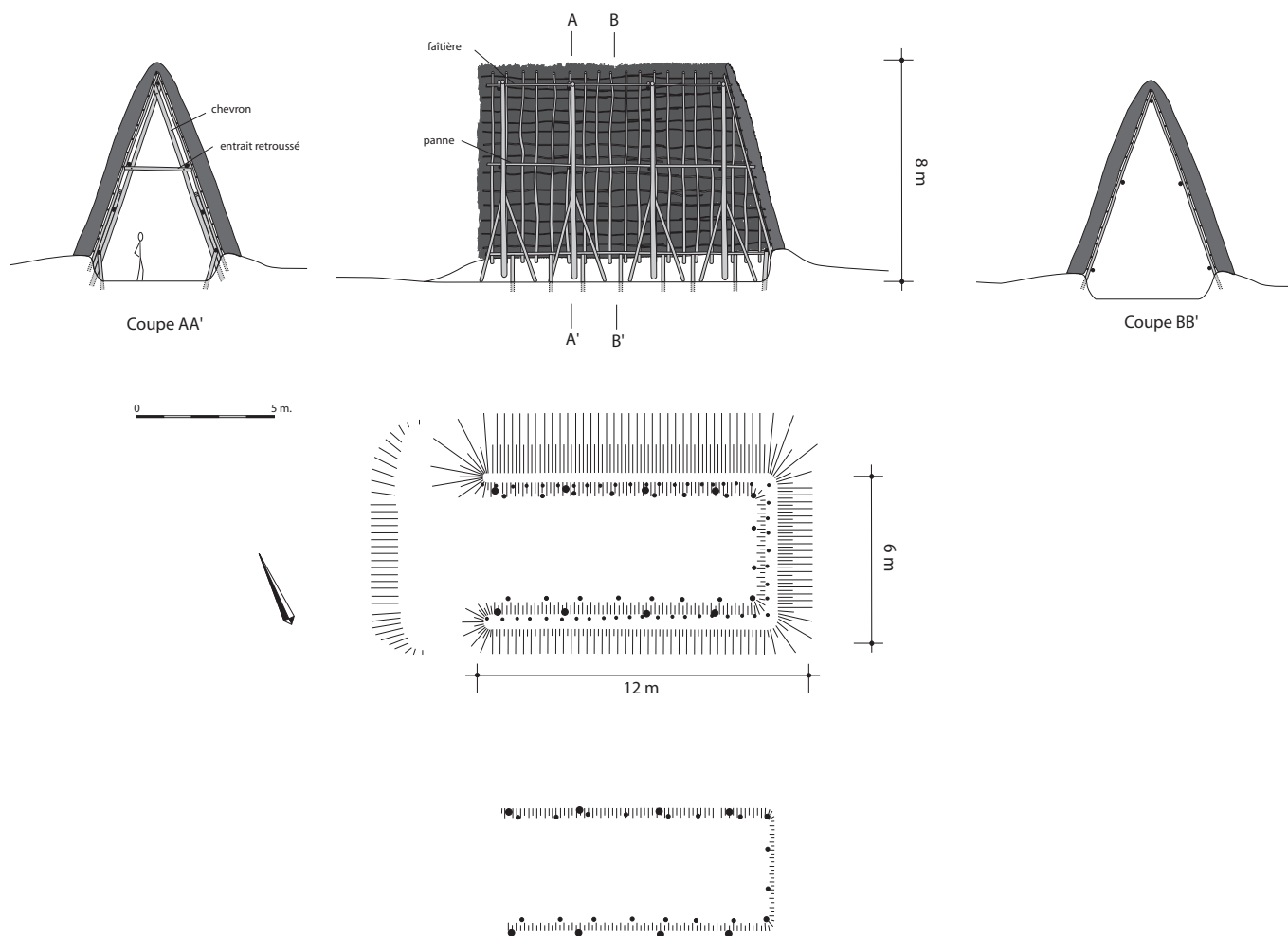
Fig. 38 Notre-Dame d'Alençon, « La Mare ». Coupes et plans (dessin F. É.).
