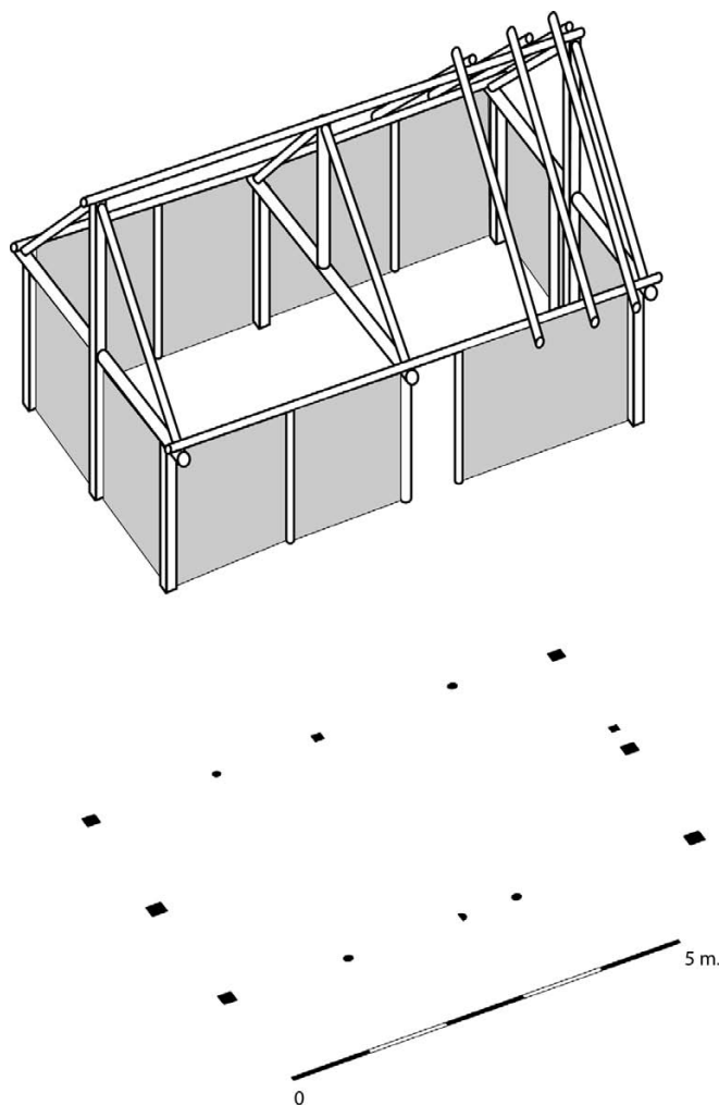
Fig. 22 Proposition de restitution d'après les traces au sol.
