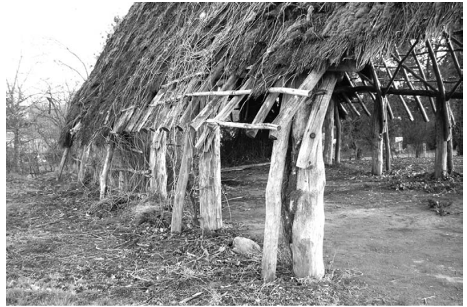
Fig. 44 Vihiers, « La Dauphinerie ». Poteaux plantés contrebutés (cl. F. É.).
