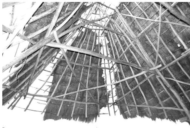
Fig. 47 Vihiers, «La Dauphinerie». Croupe débordante (cl. F. É.).
