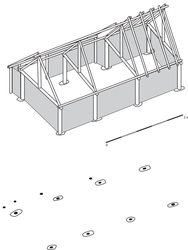
Fig. 33 Proposition de restitution d'après les traces au sol.
