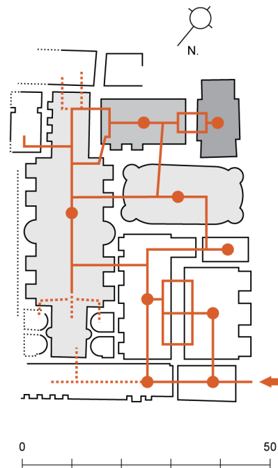
Fig. 17 – Plan typologique des bains de Hamat Gader (d'après HIRSCHFELD 1997, revu dans BROISE 2003).
