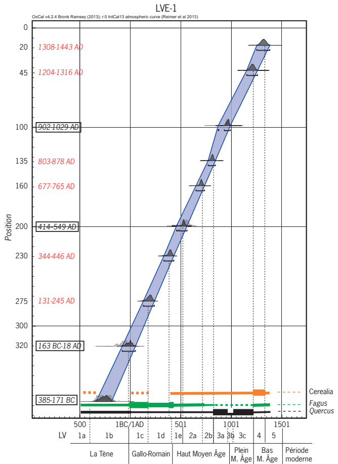
Figure 3. L'aurière de La Verrerie, dite de « Parc d'Or » (Villosanges). Modèle âge-profondeur de la carotte LVE-1 (DAO J. Argant).
