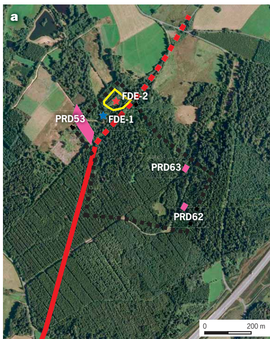
Figure 4. La zone minière de la Forêt domaniale de l'Éclache (Prondines). a : Périmètre de la zone minière avec localisation de la tourbière (jaune), du forage FDE-1, du carottage FDE-2, du tracé de la voie romaine (rouge) et des sites gallo-romains (rose) (DAO F. TRÉMENT – Géoportail - IGN) ; b : Exemple de « terrain chahuté » ; c : Vue de la tourbière depuis l'ouest.
