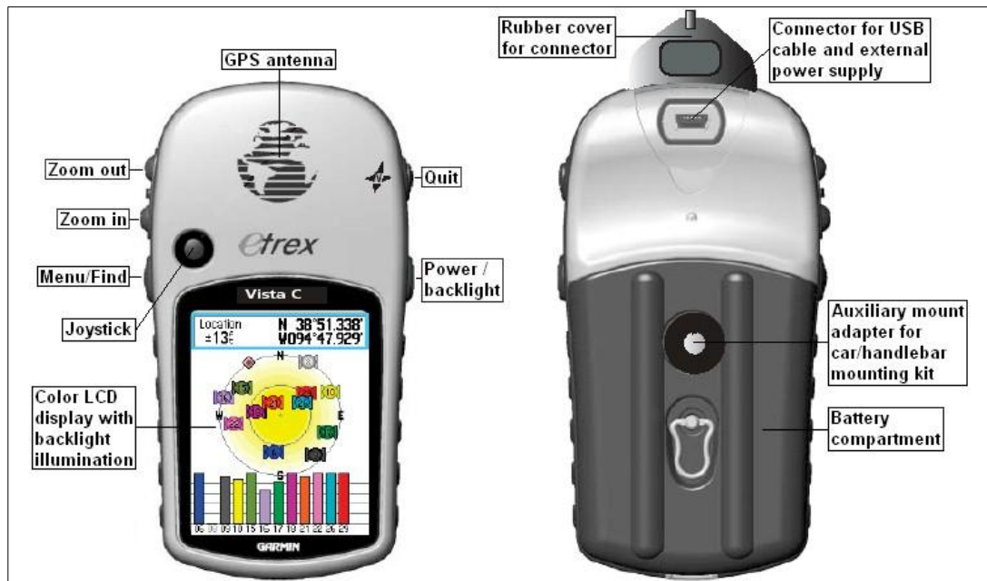
Figure 1. Schéma du boîtier GPS utilisé dans le cadre de la présente étude
