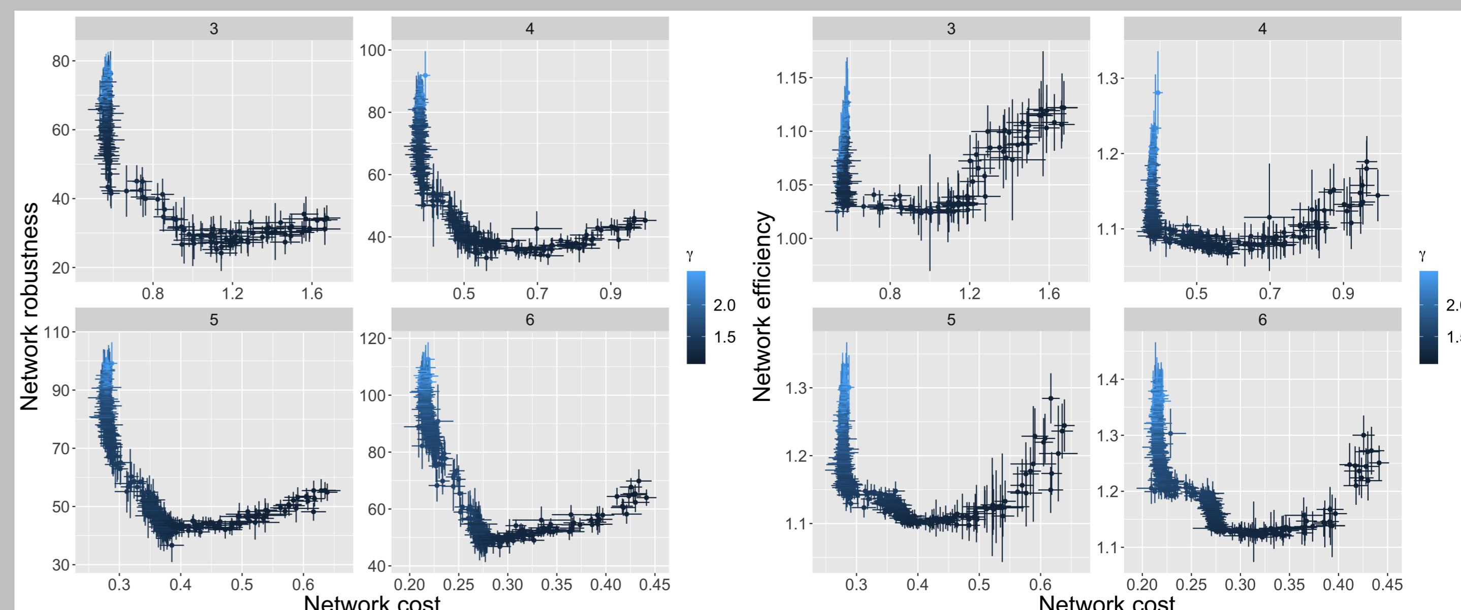
Optimisation de Pareto : fronts bi-objectifs entre les couples d'indicateurs obtenus pour un échantillonnage de 1000 valeurs pour \gamma , nombre de centres de 3 à 6 (sous-graphes) et 100 répliques (barres d'erreurs : intervalles de confiance à 95%).
