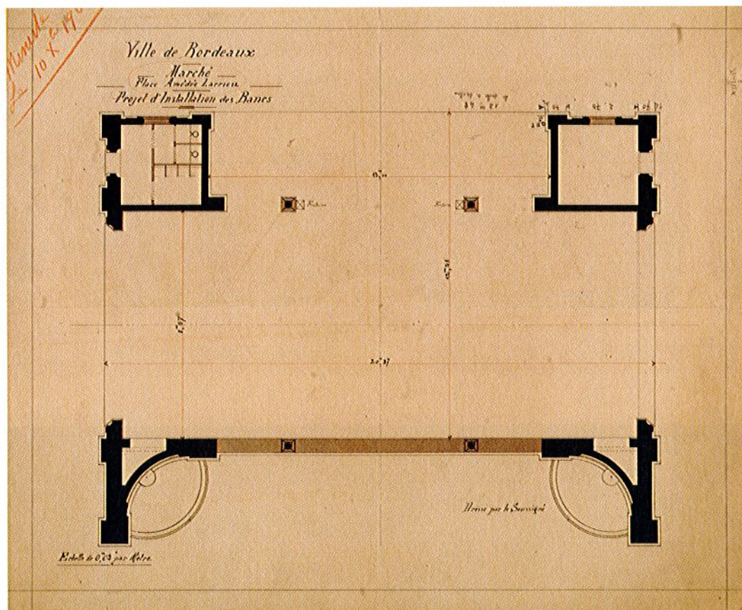
Fig. 6. - Plan du marché couvert pour installation des banes, 10 décembre 1901, A.M.Bx, cote 139 M 4. Cl. Bernard Rakotomanga.
