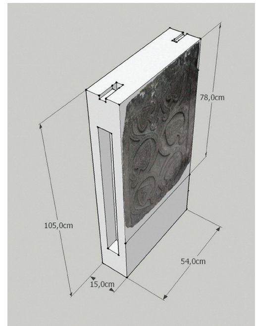
Fig. 9 – Restitution du pilier de chancel de la fig. 7 (cl. et DAO J. Crochat)
