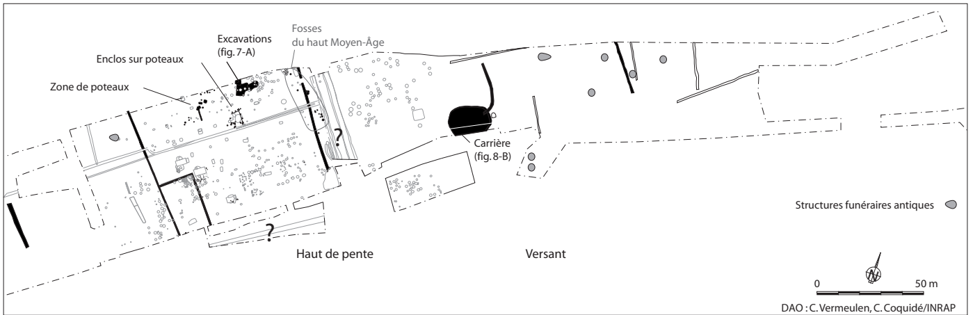
Fig. 6△. Meyzieu "La Chapelle" et "Les Hermières" : plan masse.
