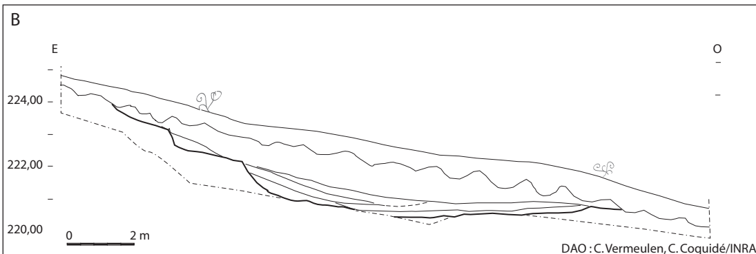
Fig. 8▽. Meyzieu "La Chapelle" et "Les Hermières" : carrière, coupe.
