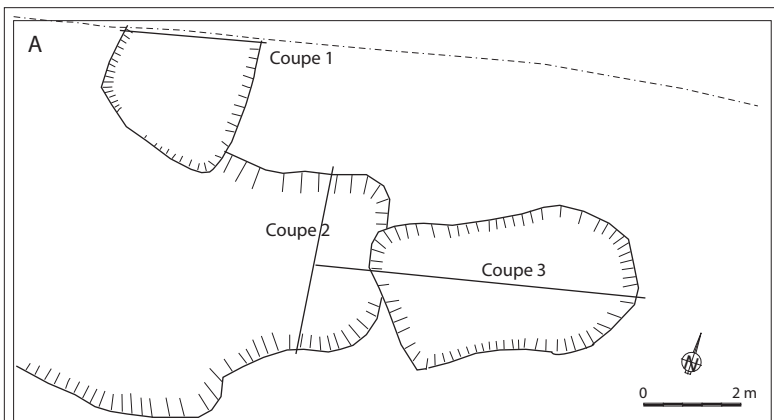
Fig. 6△. Meyzieu "La Chapelle" et "Les Hermières" : plan masse.
