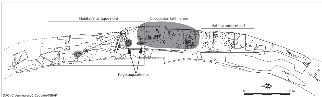
Fig. 5. Chassieu-Genas "L'Épine" : plan masse et évolution (Coquidé & Vermeulen 1999).
