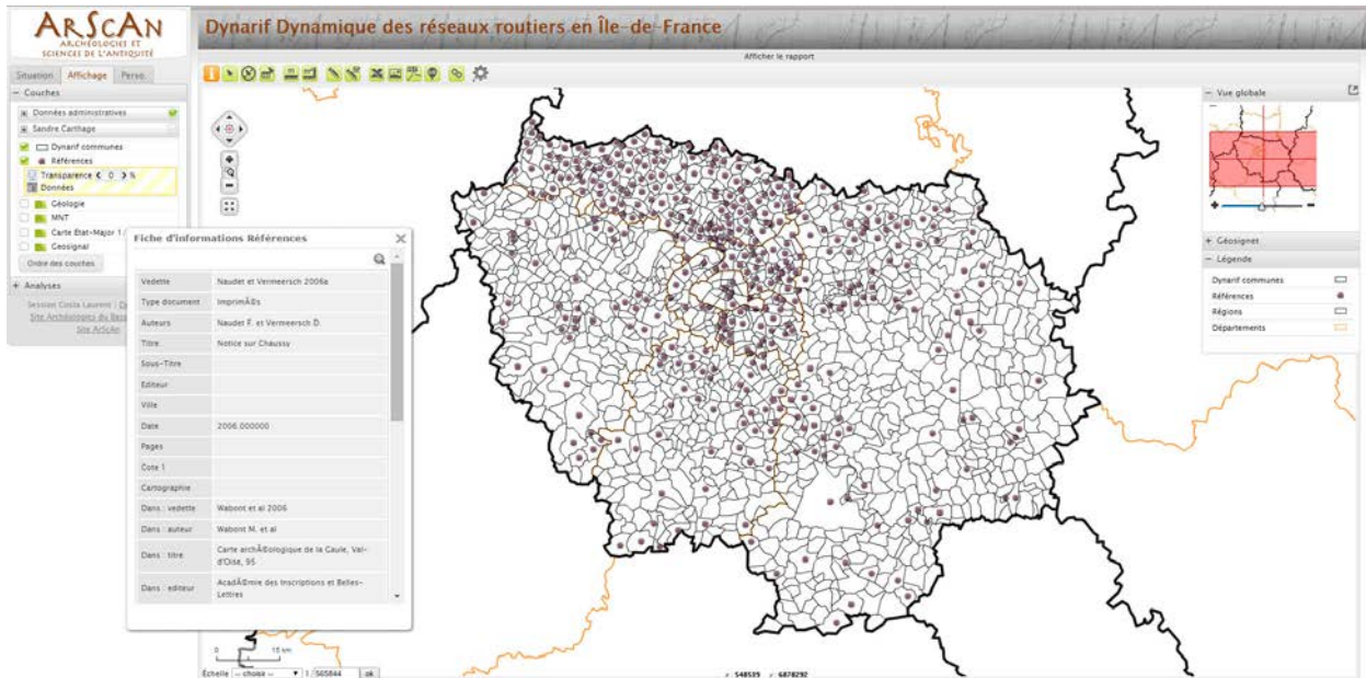
Figure 1 : L'interface Reagit-Dynarif.
