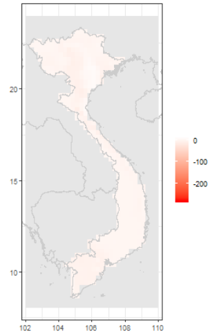
(d) RCP8.5 - 2050
