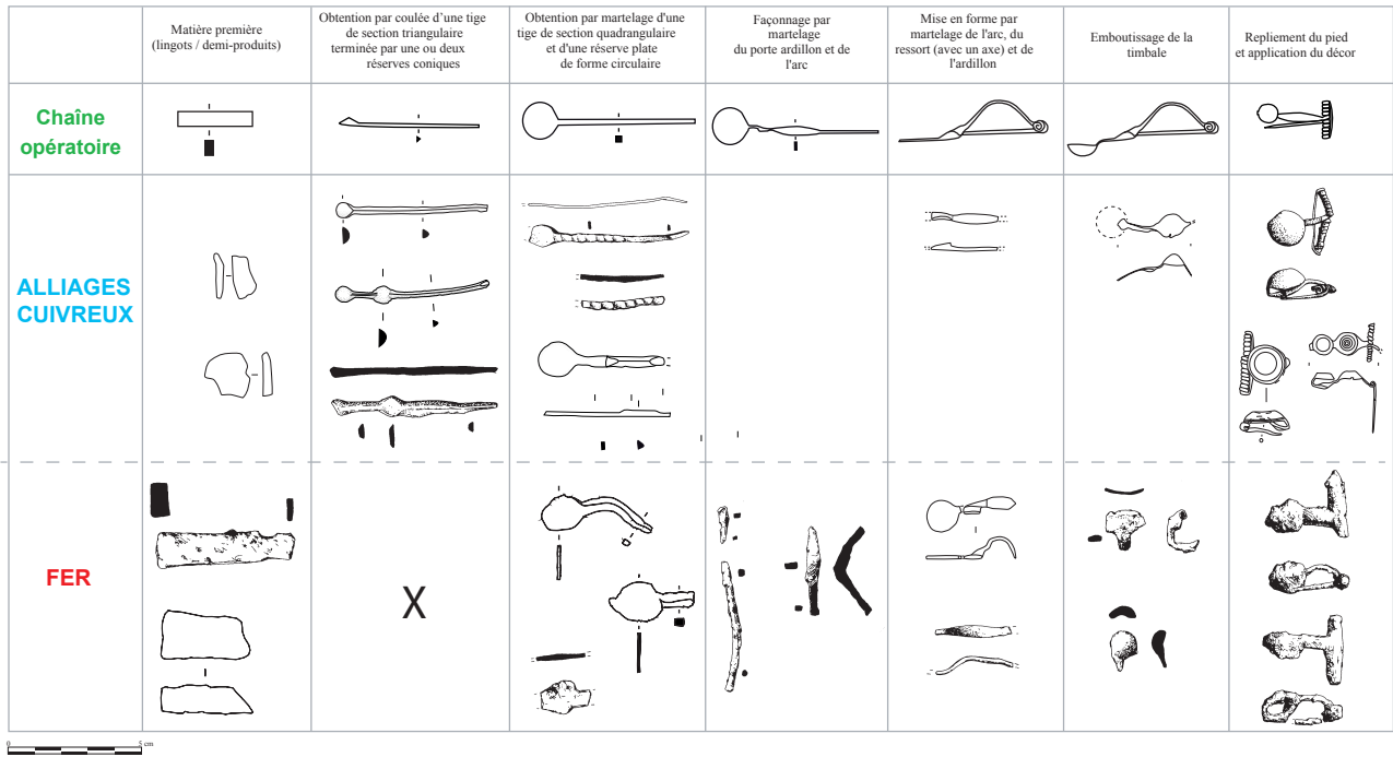
Fig. 5 – Chaîne opératoire de la fabrication des fibules à timbale en fer et bronze (D'après Cararra et al. , 2013, fig. 4 ; DAO E. Dubreucq).
