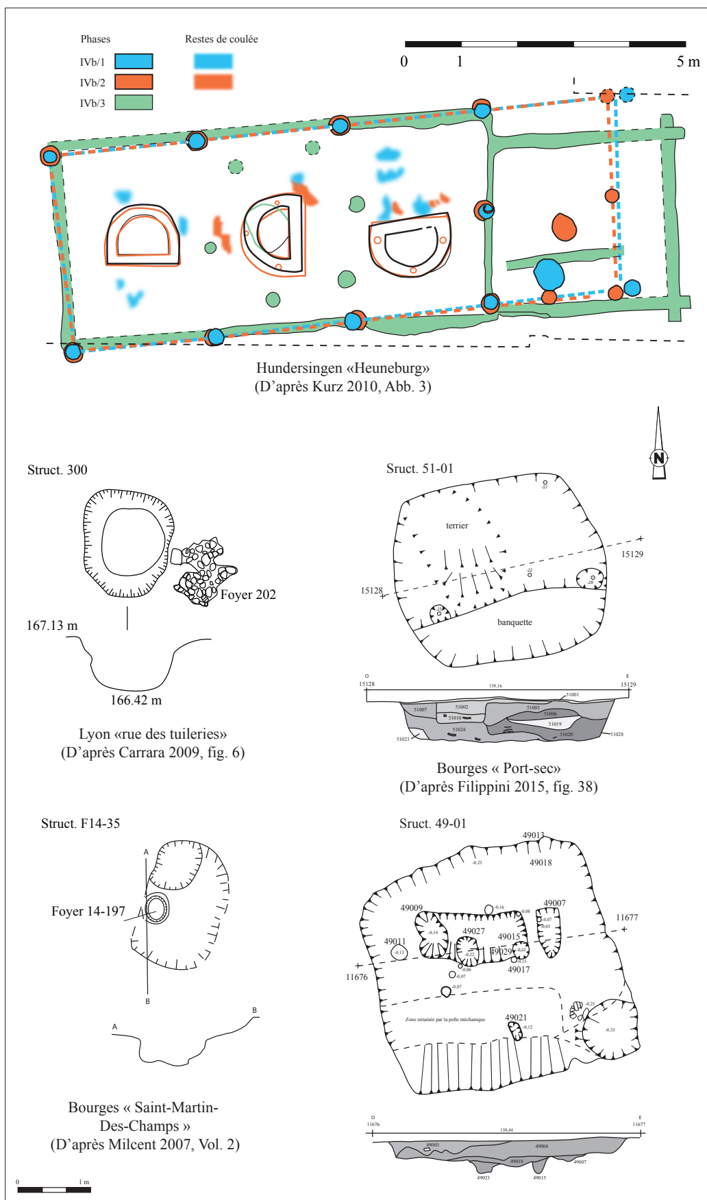
Fig. 2 – Exemples de structures d’ateliers : celui de la Heuneburg (Bade-Wurtemberg) et les fosses-ateliers typiques du Ha D3-LTA1 à Lyon et Bourges (France ; DAO E. Dubreucq). Fig. 2 – Examples of workshops: Heuneburg (Baden-Württemberg) and typical pit-workshop dated of Ha D3-LTA1 at Lyon and Bourges (France; CAD E. Dubreucq).
