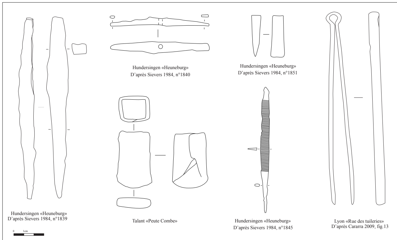
Fig. 3 – Quelques outils de métallurgistes trouvés sur les habitats entre la fin du VI e et le début du V e siècle avant notre ère (DAO E. Dubreucq).
