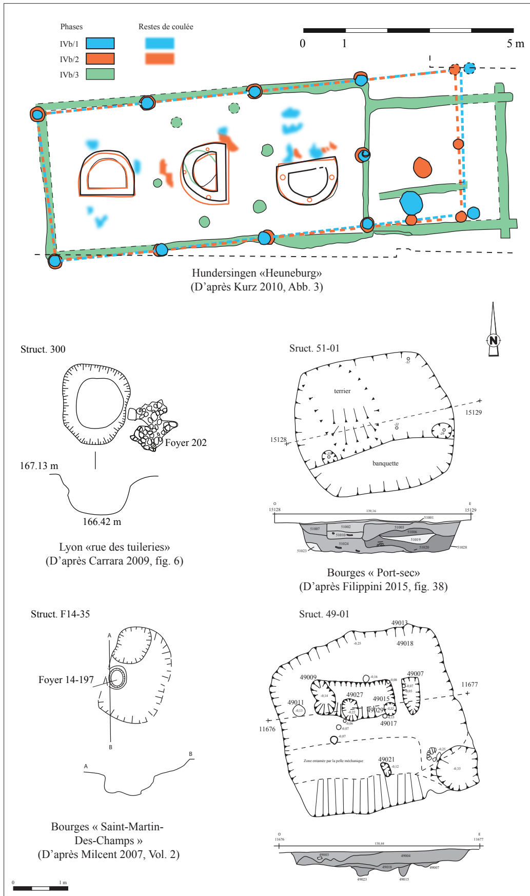
Fig. 2 – Exemples de structures d’ateliers : celui de la Heuneburg (Bade-Wurtemberg) et les fosses-ateliers typiques du Ha D3-LTA1 à Lyon et Bourges (France ; DAO E. Dubreucq). Fig. 2 – Examples of workshops: Heuneburg (Baden-Württemberg) and typical pit-workshop dated of Ha D3-LTA1 at Lyon and Bourges (France; CAD E. Dubreucq).
