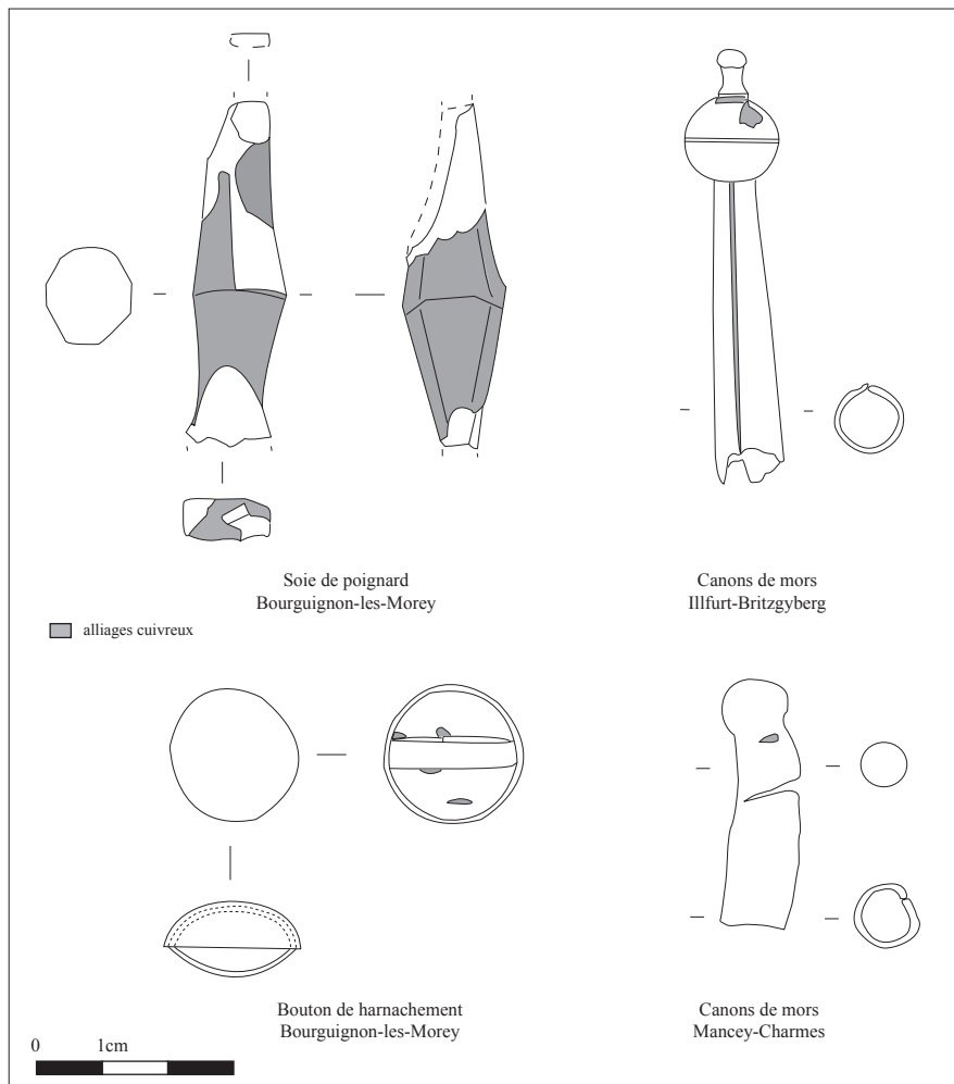
Fig. 8 – Quelques-uns des objets en fer ayant bénéficié de brasure (Dessin et DAO E. Dubreucq, d'après Dubreucq, 2013). Fig. 8 – Examples of fews iron objects with brazing (Drawing & CAD E. Dubreucq, after Dubreucq, 2013).
