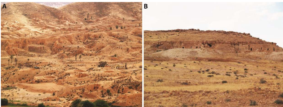
Figure 8. Habitations troglodytiques creusées dans la couverture loessique, entre Chemlali et Sidi Meta (A) et dans un banc de calcaire tendre à Ksar Hadada (B)
