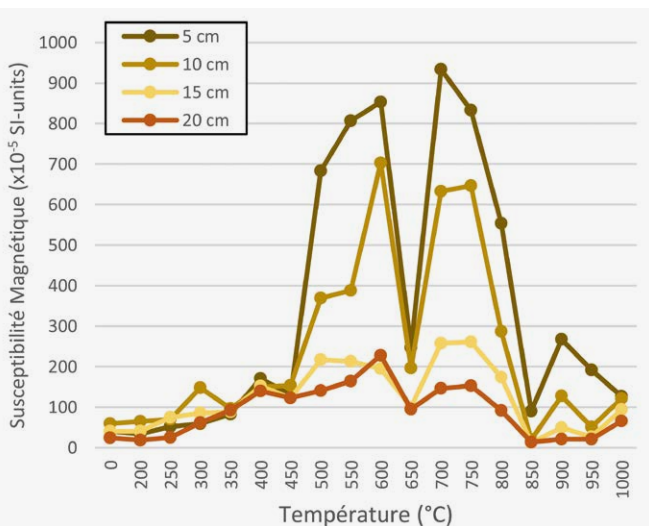
Figure 9. Evolution de la susceptibilité magnétique en fonction des températures de chauffe des échantillons de terre fine de différentes profondeurs.
