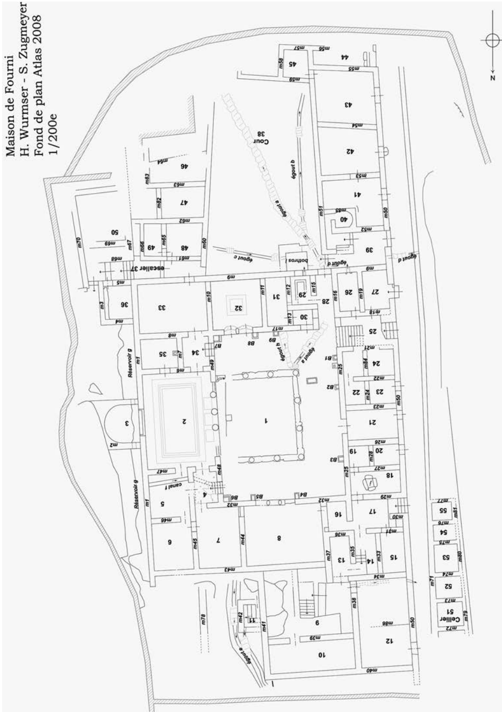
1. Plan de la Maison de Fourni. Fond de plan relevé en 2008, Atlas de Délos, EAD XLIII, ÉfA, 2015. Compléments et numérotation St. Zugmeyer et H. Wurmser.
