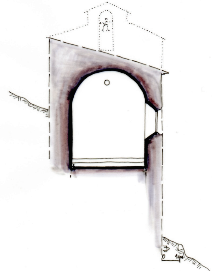
Chapelle Saint- Roch (Les Mées) schémas de principe
