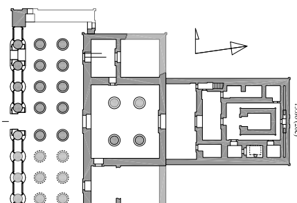
Temple d'Isis, Chenhour (Auguste, Tibère, Trajan) d'après Dilis, Traunecker
