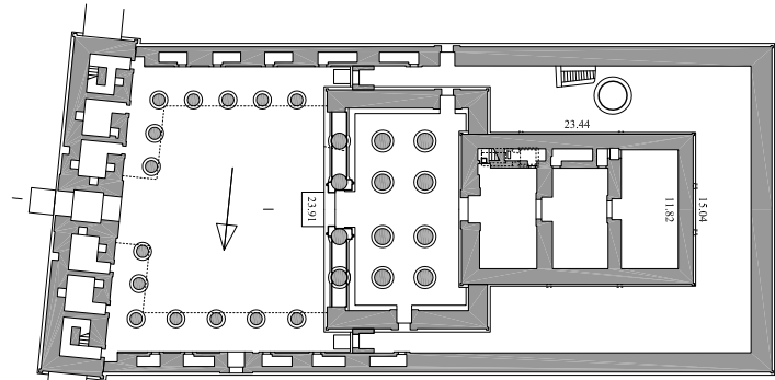
Temple de Mandoulis et Isis, Kalabcha (Auguste) d'après Steigler 1970
