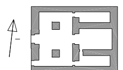
Temple d'Isis, Assuan (Ptolémée III) d'après Von Pilgrim 2006
