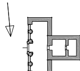
Temple de Khnoum, Satet et Anuket, Assuan (Domitien) d'après Jaritz 1975
