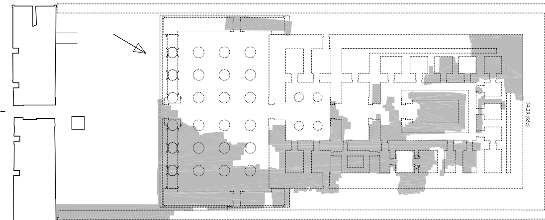
Temple de Montou, Ermant (Ptolémée XII) d'après Zignani 2014
