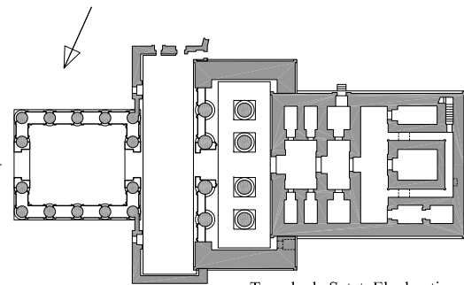
Temple de Satet, Elephantine (Ptolémée VI, VIII) d'après Ricke 1960
