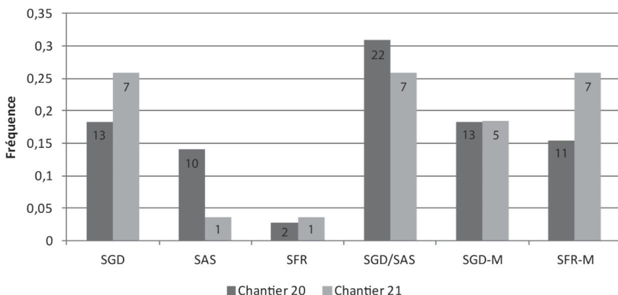
Fig. 3.11 Représentation des différents faciès de scorie au sein du corpus de culots de forge (A. Dissler).
