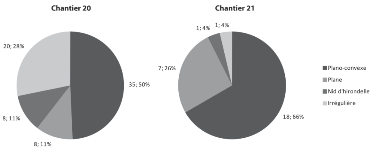
Fig. 3.8 Proportions des sections de scories en calotte (A. Dissler).
