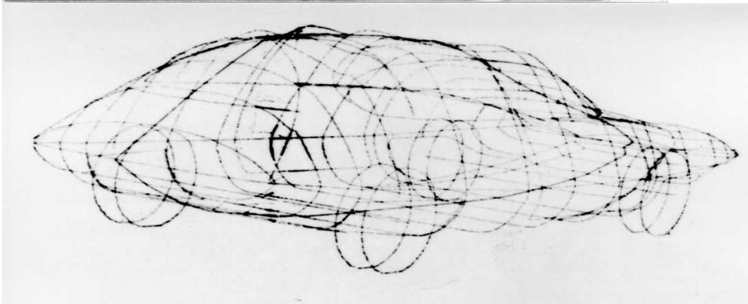
Croquis de carrosserie en CAO par le système Unisurf, 1964
