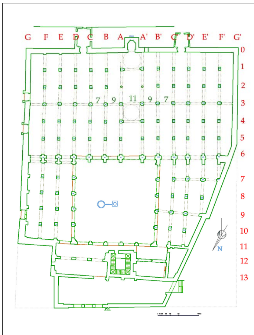
fig. 1 - Plan de la grande mosquée de Taggart et numérotation des travées. (Institut méditerranéen)
