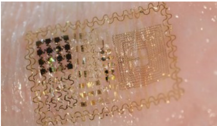
Maille nanométrique dotée de capteurs, l'Université de Tokyo, 2017
