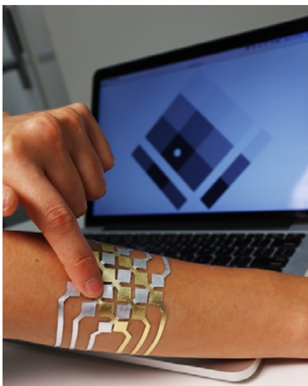
Tatouage électronique DuoSkin , MIT © Jimmy Day, 2016.
