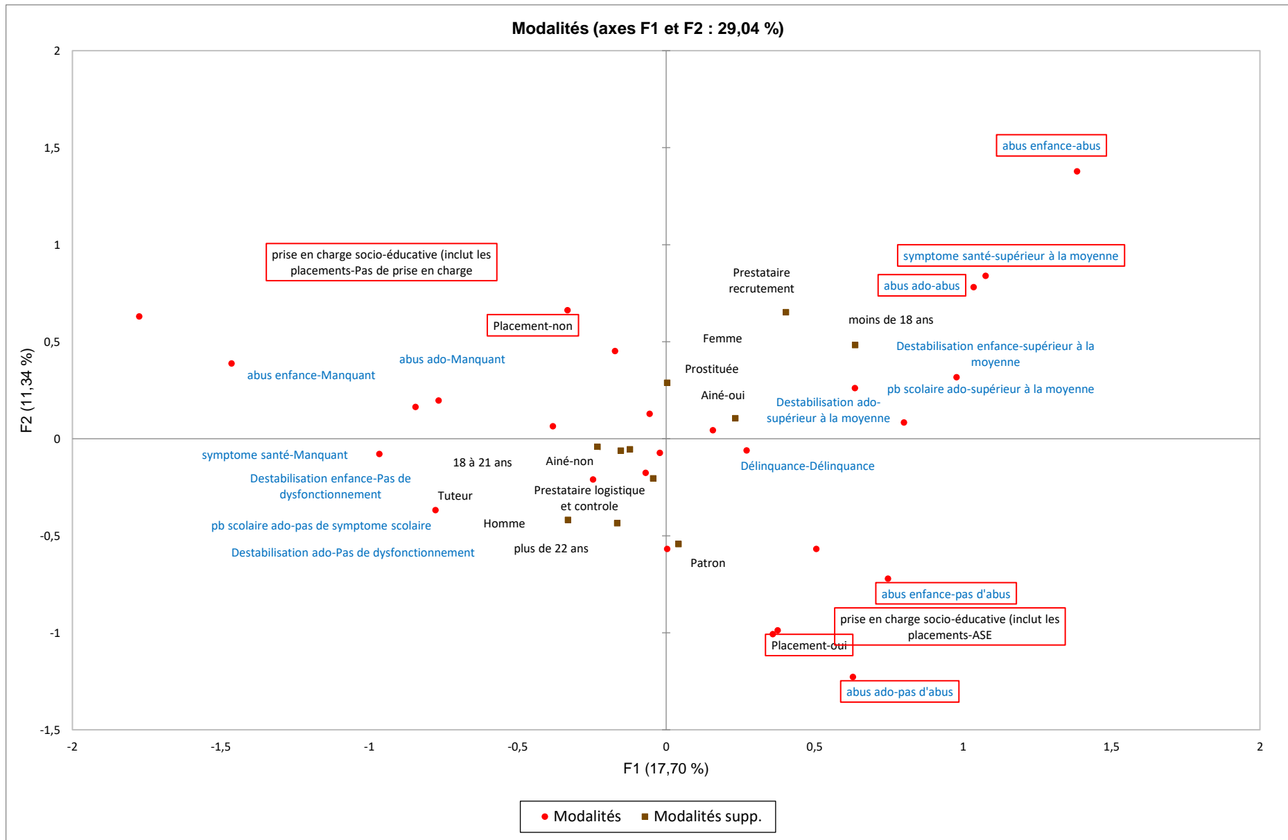
Figure 1 : Carte de l'analyse des correspondances multiples
