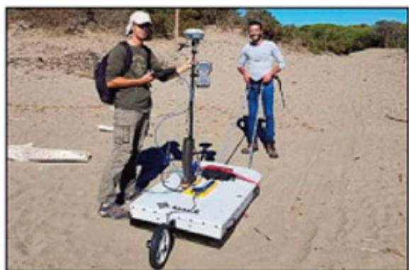
C. Géoradar sur le cordon sud
