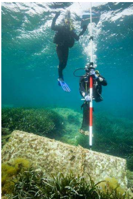
Fig. 3 : Vue sous-marine des opérateurs durant le lever topométrique
