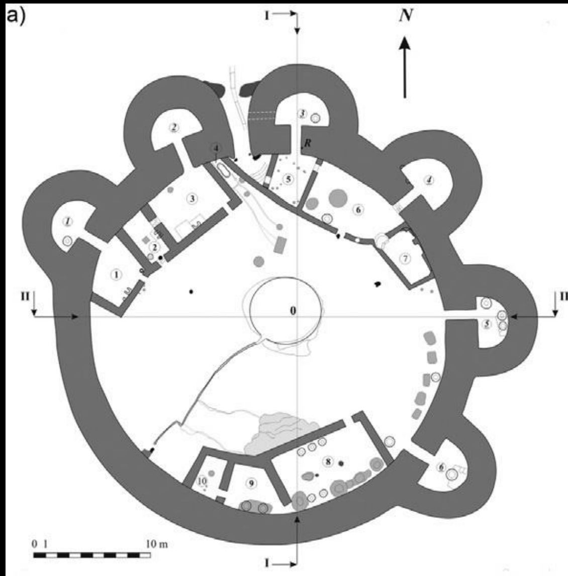
Plan de la citadelle de Kurganzol (Ouzbékistan)
