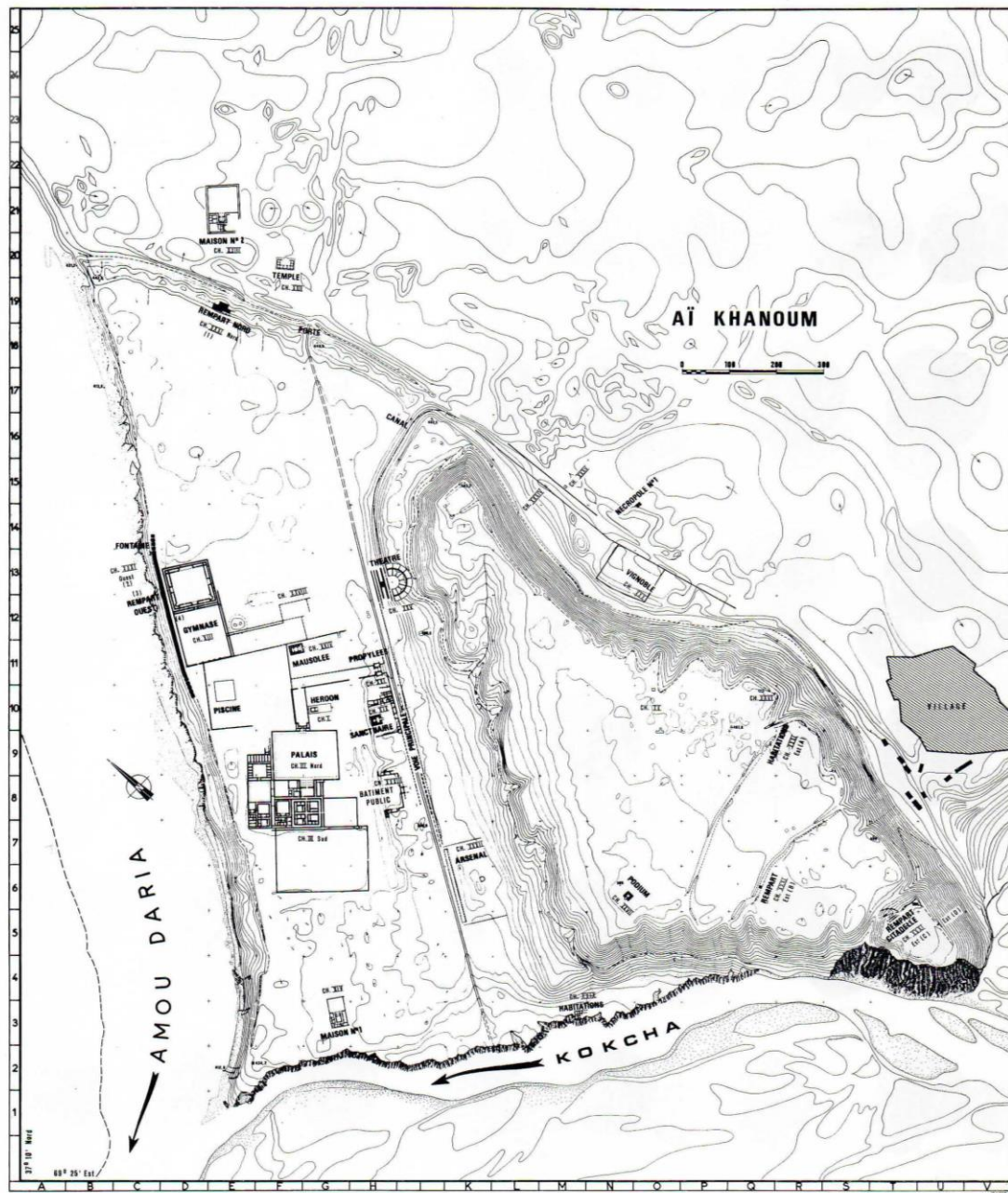
Plan du site avec les différents chantiers (dessin de J.-Cl. Liger).
